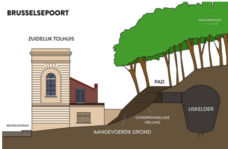
Doorsnede en ligging - actiegroep 'Red de Brusselsepoort'
